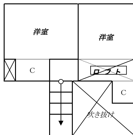
—2階平面図—
