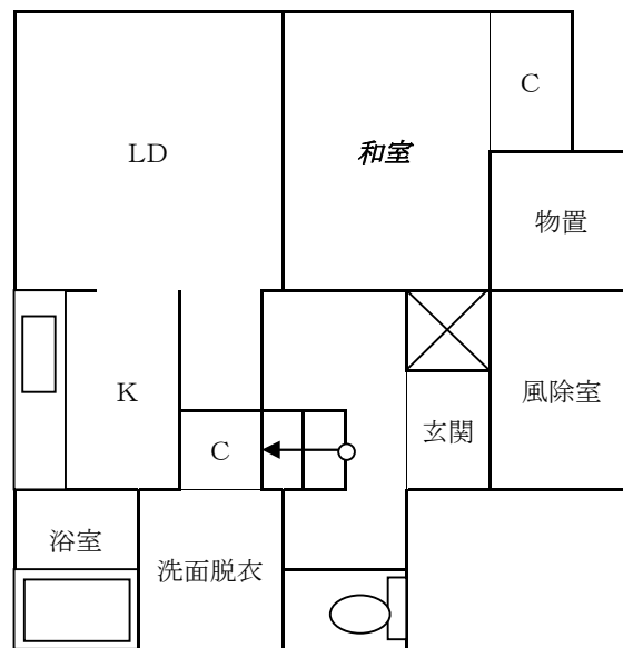
—1階平面図—
