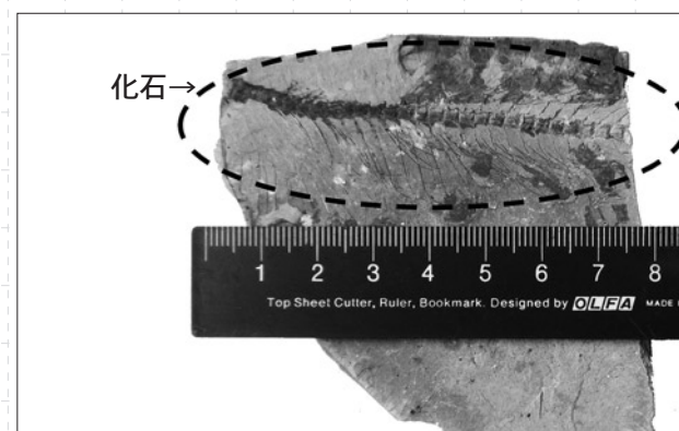
写真2 化石を含む泥岩
