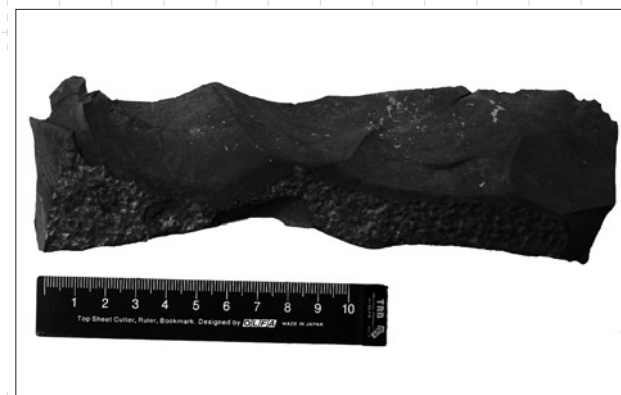
写真3 まっ黒い泥岩
